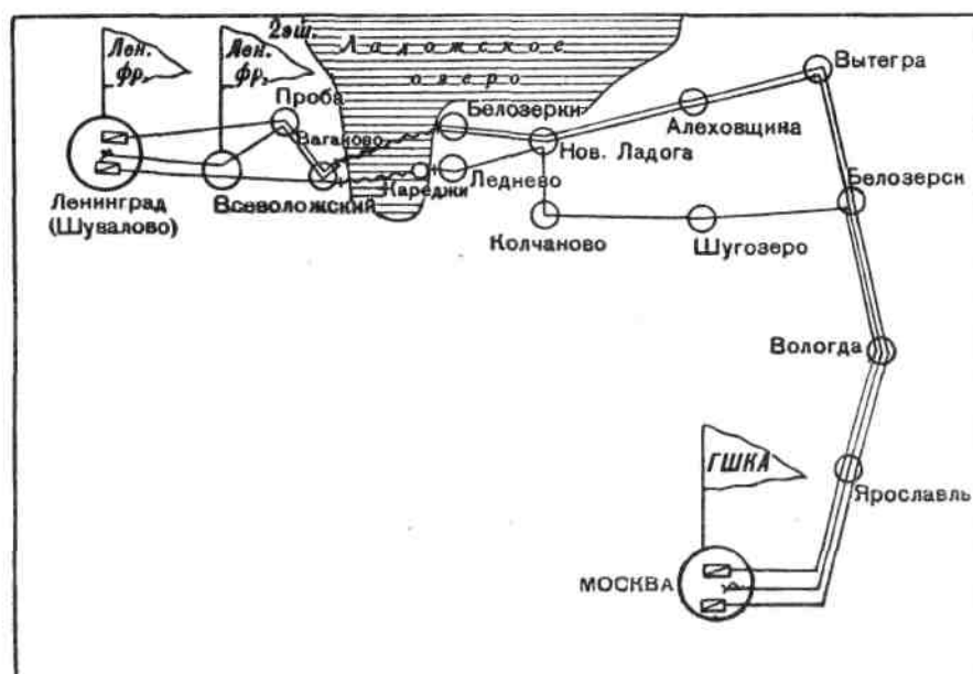
Рис.2. Проводная связь Ставки со штабом Ленинградского фронта по кабелю, проложенному по дну Ладожского озера.
